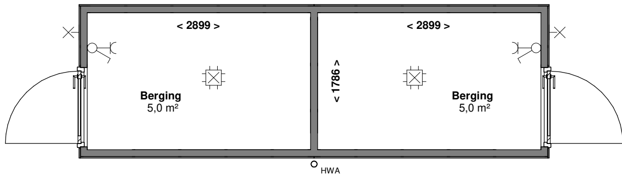
Begane grond
